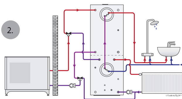
1. GTV Technik с геотермальной системой 2. GTV Technik с системой теплового насоса воздух-вода
