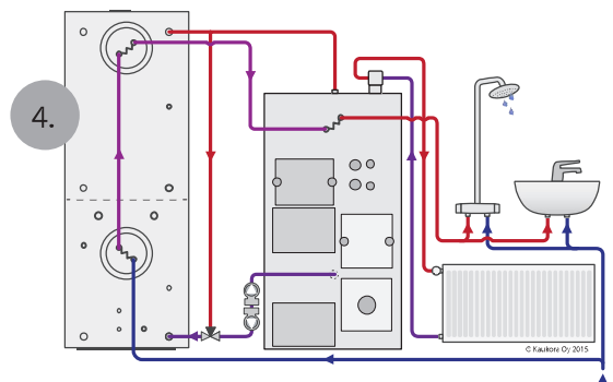
3. GTV Technik с системой солнечных коллекторов 4. GTV Technik с комбинированным котлом
